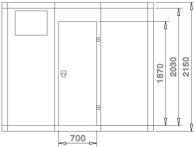
Zij aanzicht
